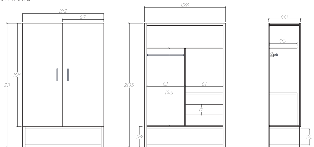
ARMARIO
