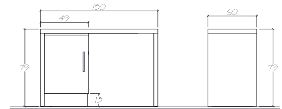
BANCO - PORTAMALETAS
